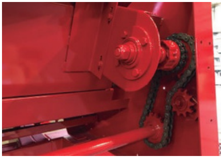
Transmisión de sinfín independiente de eje de mando de caja.
